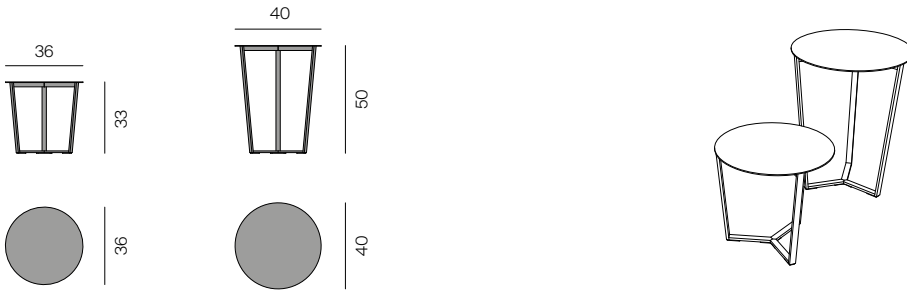
PERO Beistelltisch PERO side table
