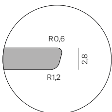
Plattenquerschnitt Cross-section tabletop
