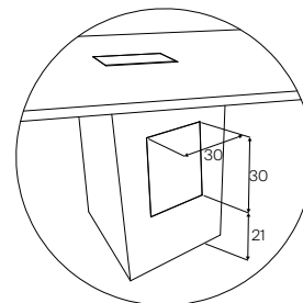
Revisionsklappe Revision flap
