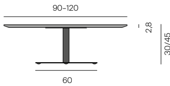
B14 Couchtisch quadratisch B14 coffee table square
